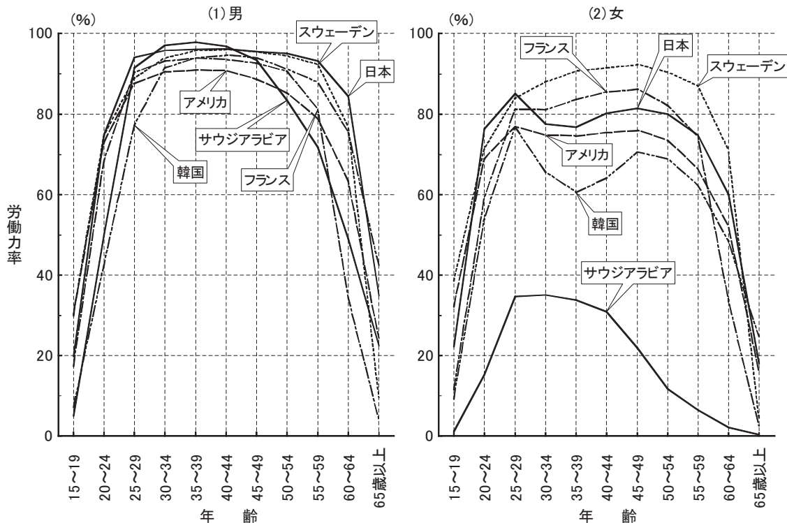
図8-5 主要国の性、年齢別労働力率：2019年
