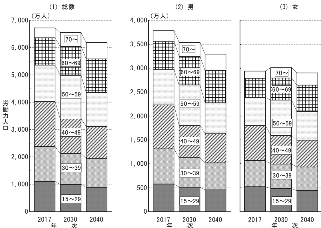
図 8-4 性、年齢別労働力人口の将来推計：2017～40年
