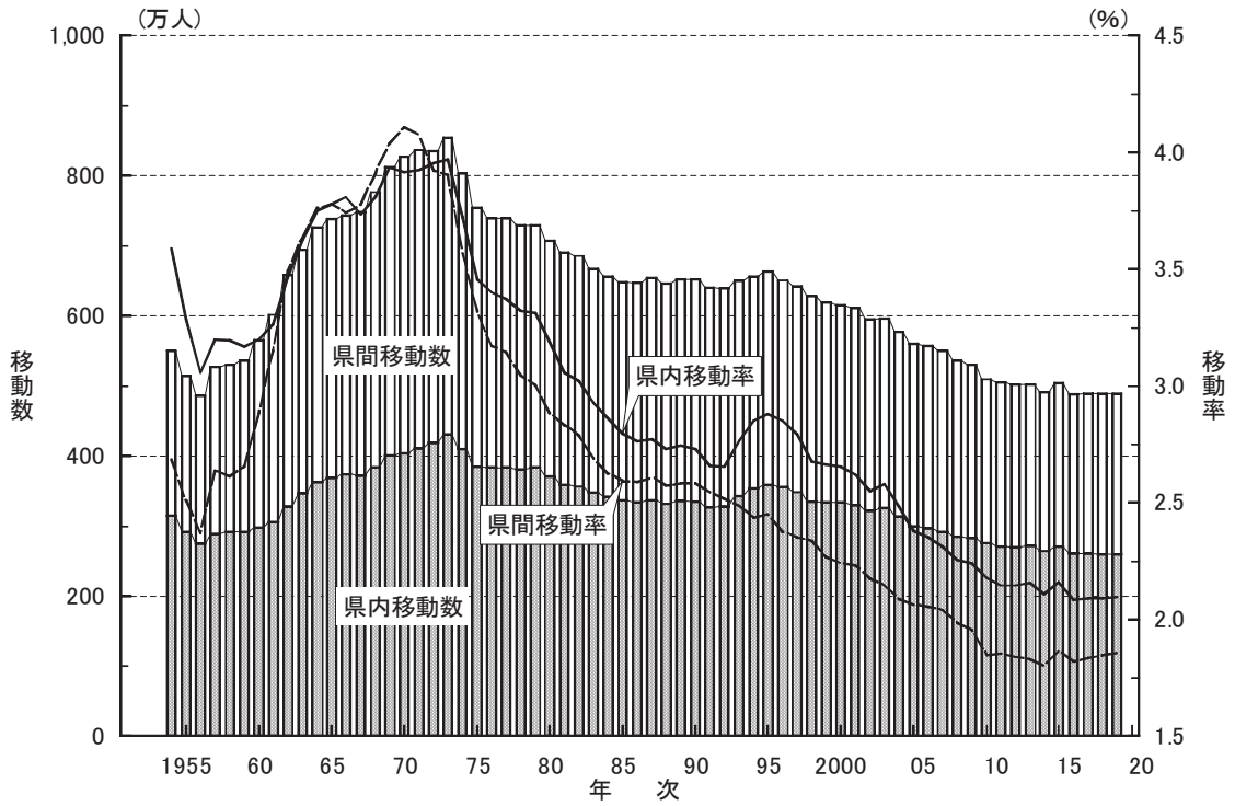
図9-1 県内・県間別人口移動数および率：1954～2019年
