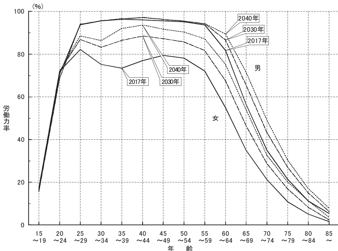
図8-3 性、年齢別労働力率の将来推計：2017～40年
