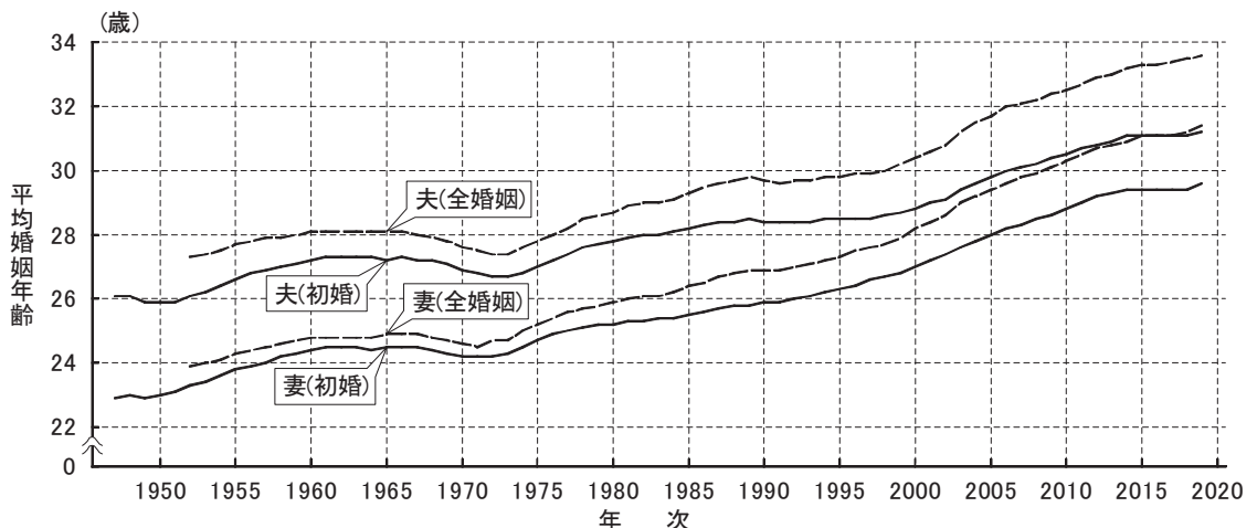
図6-4 全婚姻および初婚の平均婚姻年齢：1947～2019年
