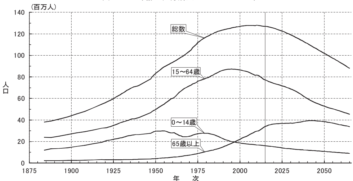
図2-2 年齢3区分別人口：1884～2065年
