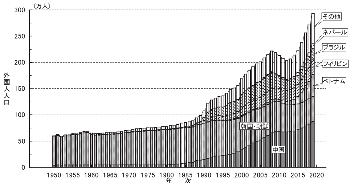
図 10-1 国籍別在留外国人人口：1950～2019年
