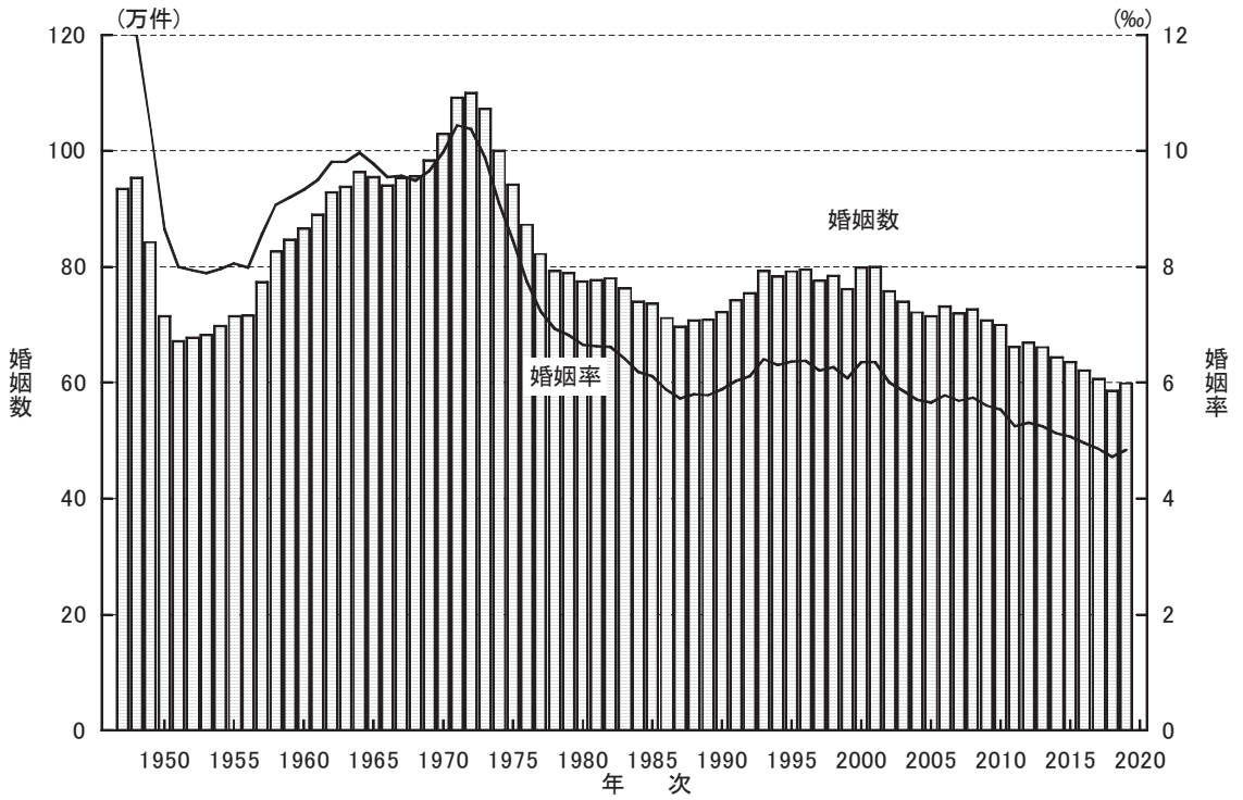
図 6 - 1 婚姻数および婚姻率：1947～2019年
