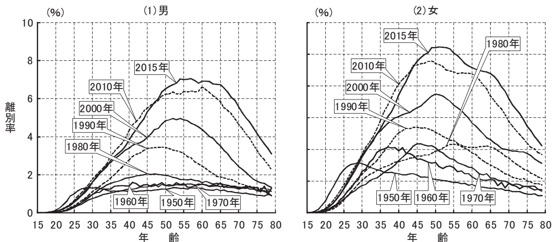
図6-5-4 性、年齢別離別割合：1950～2015年
