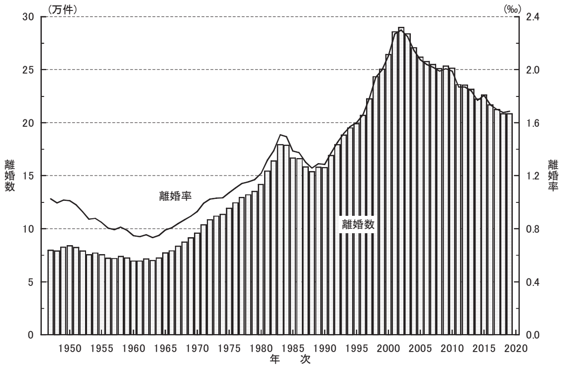
図 6 - 2 離婚数および離婚率：1947～2019年
