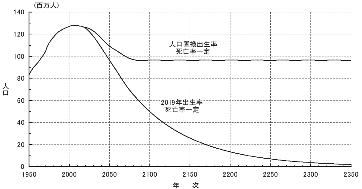
図3-2 2019年以降出生率, 死亡率一定による人口総数
