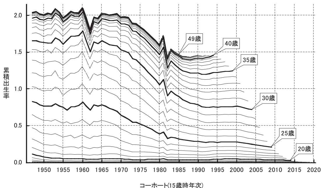
図4-5 女性のコーホート別累積出生率：1947～2019年コーホート
