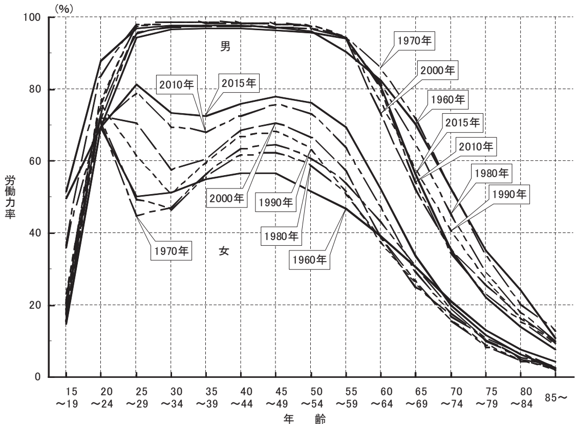
図 8-2 性、年齢別労働力率：1960～2015年
