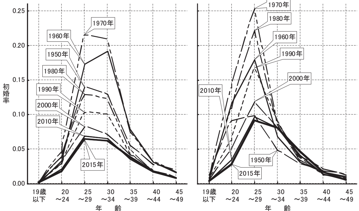
図6-3 未婚者に対する初婚率：1950～2015年
