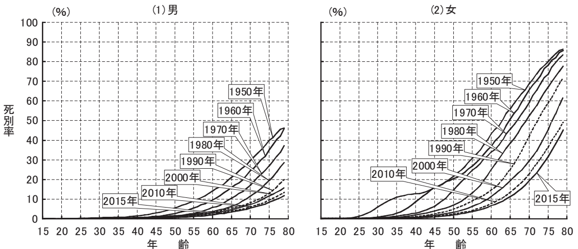
図6-5-3 性、年齢別死別割合：1950～2015年
