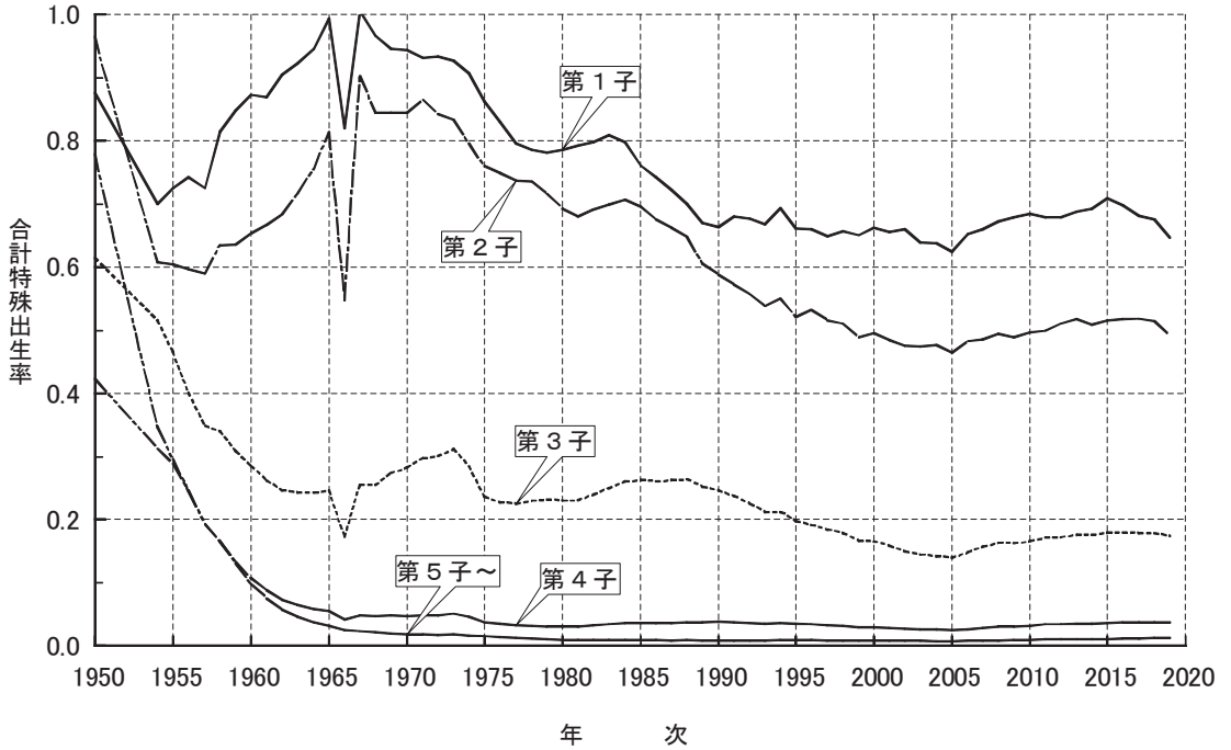
図4-6 出生順位別合計特殊出生率：1950～2019年
