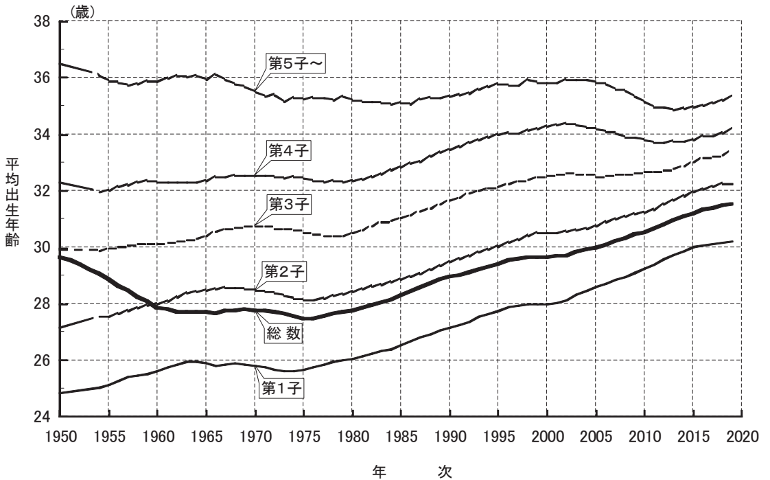
図4-7 出生順位別平均出生年齢：1950～2019年
