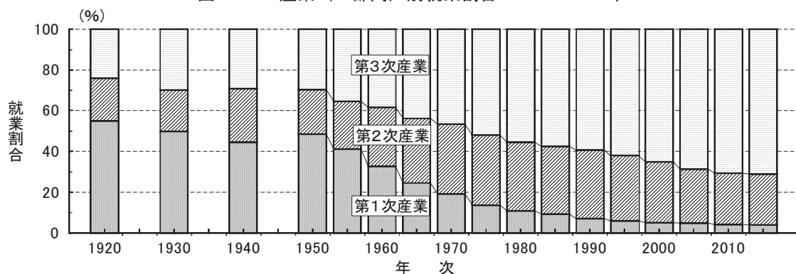
図8-6 産業（3部門）別就業割合：1920～2015年
