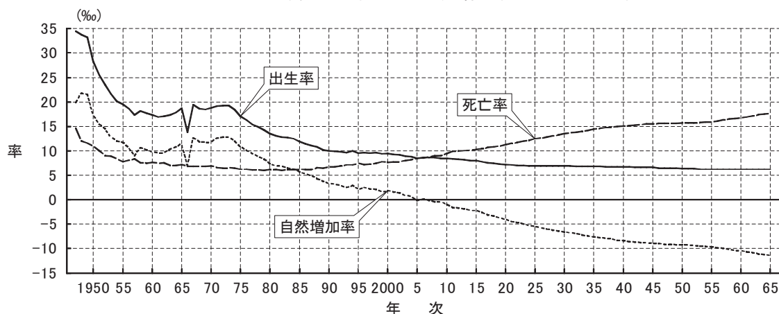
図3-1 出生率、死亡率および自然増加率：1947～2065年
