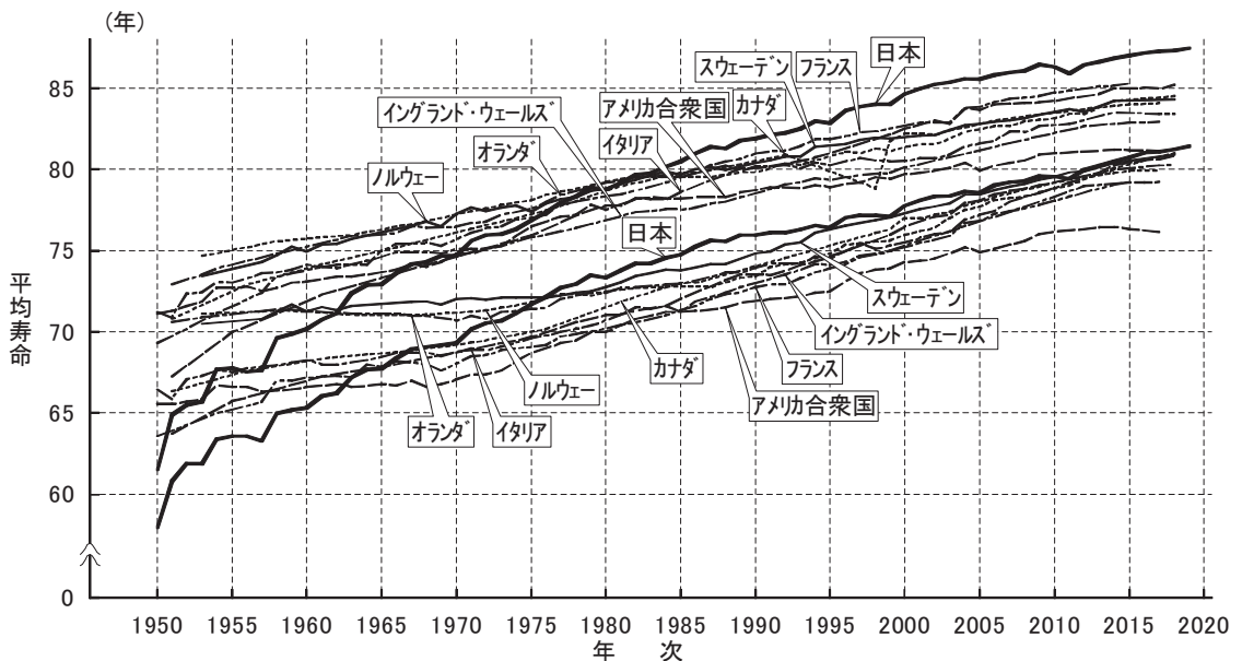
図5-3 主要国の平均寿命：1950年～最新年次
