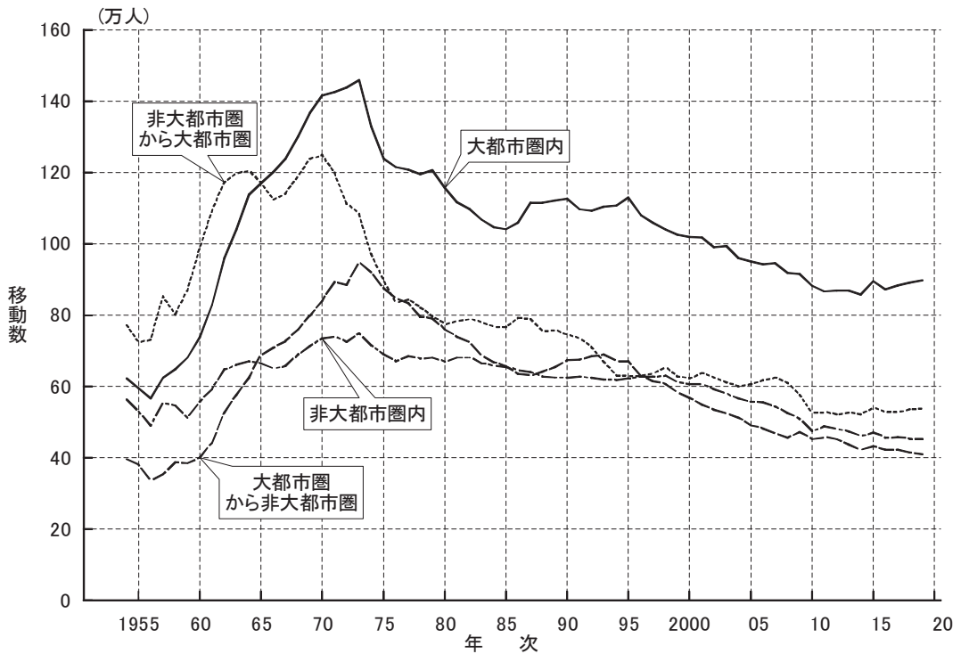
図9-2 類型別県間移動数：1954～2019年
