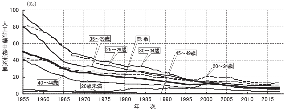
図4-8 年齢別人工妊娠中絶実施率：1955～2018年
