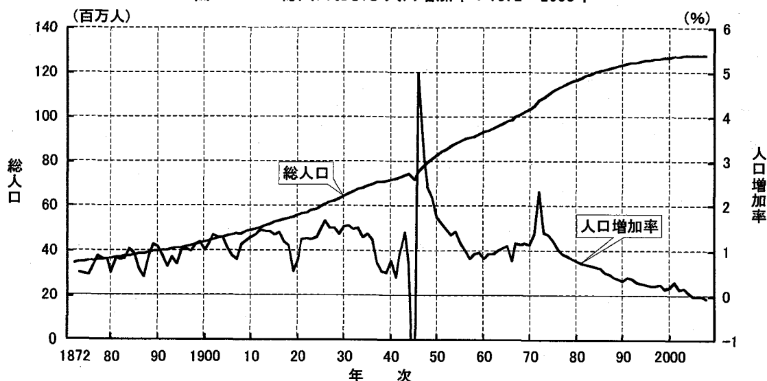
図1-1 総人口および人口増加率：1872～2008年
