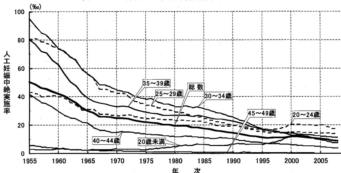
図4-9 年齢別人工妊娠中絶実施率：1955～2008年
