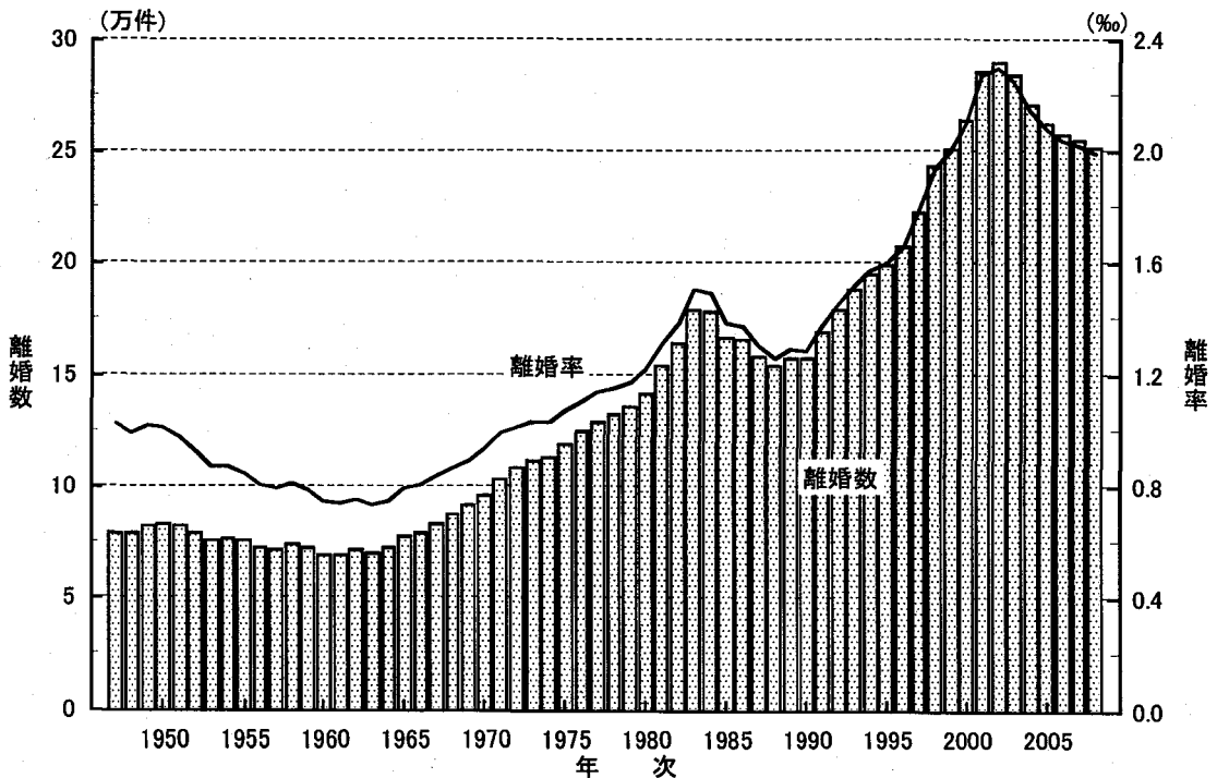
図 6 - 2 離婚数および普通離婚率：1947～2008年
