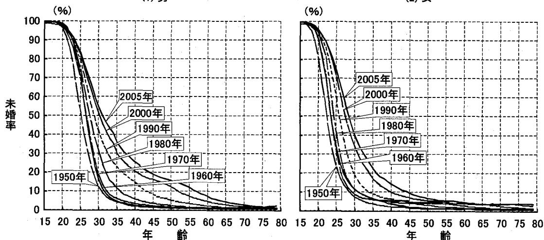
図6-5-1 性、年齢別未婚率：1950~2005年
