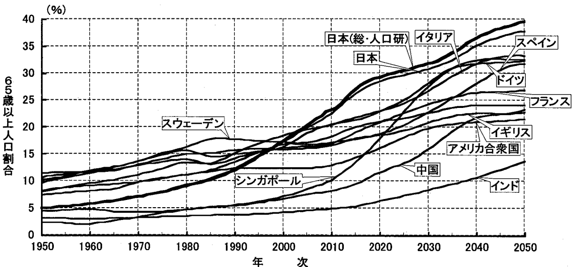
図2-4 主要国の65歳以上人口割合：1950～2050年
