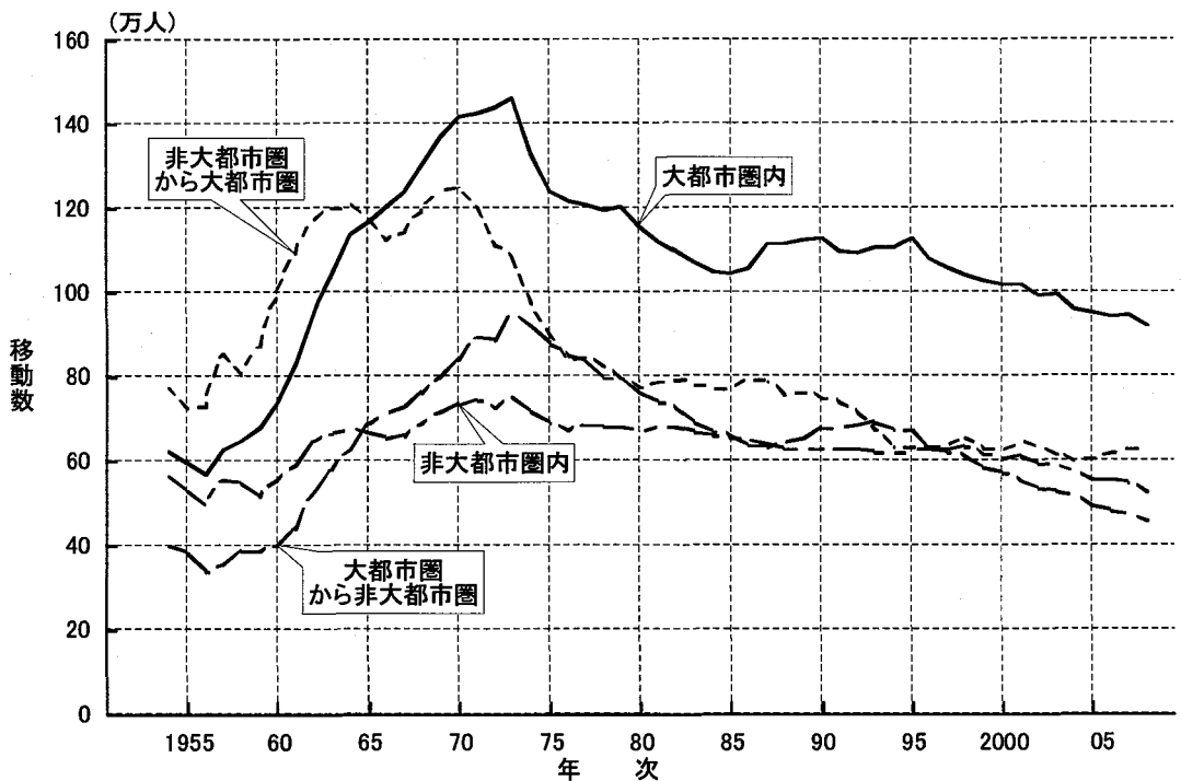
図9-2 類型別県間移動数：1954~2008年
