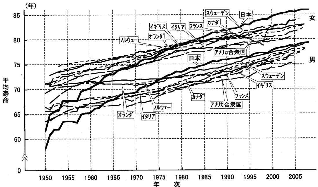
図5-3 主要国の平均寿命：1950年～最新年次
