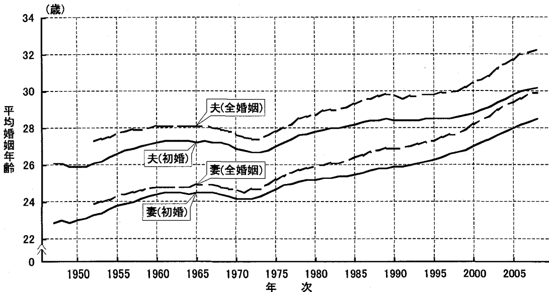
図6-4 全婚姻および初婚の平均婚姻年齢：1947～2008年
