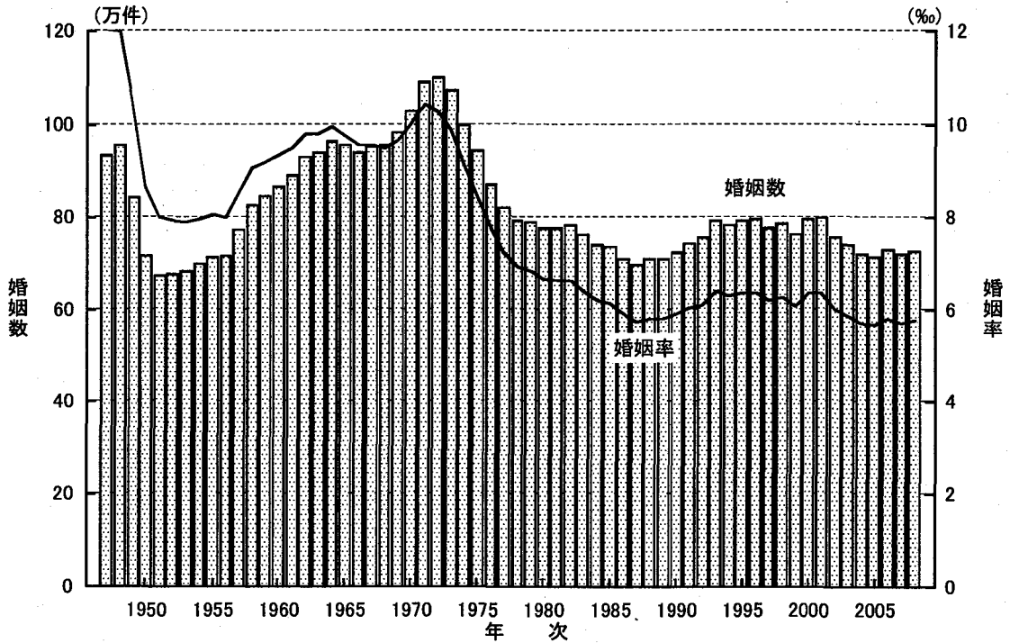
図 6 - 1 婚姻数および普通婚姻率：1947～2008年
