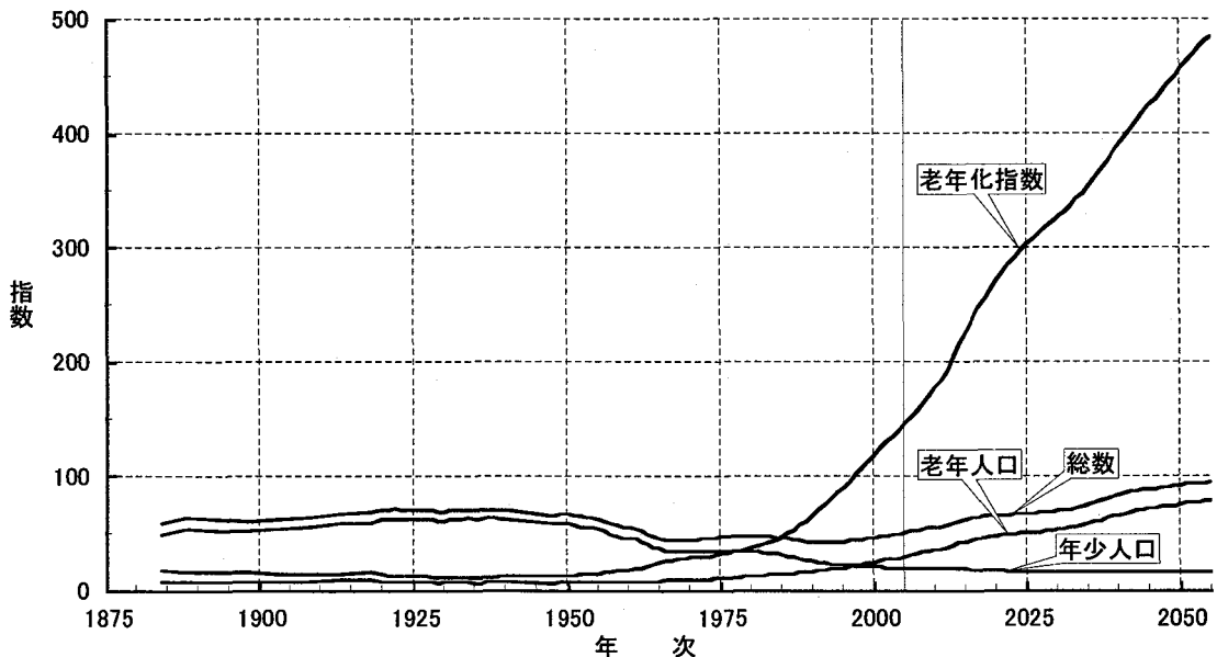
図2-3 従属人口指数および老年化指数：1884～2055年
