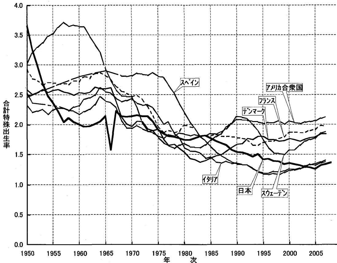
図4-2 主要先進国の合計特殊出生率：1950年～最新年次
