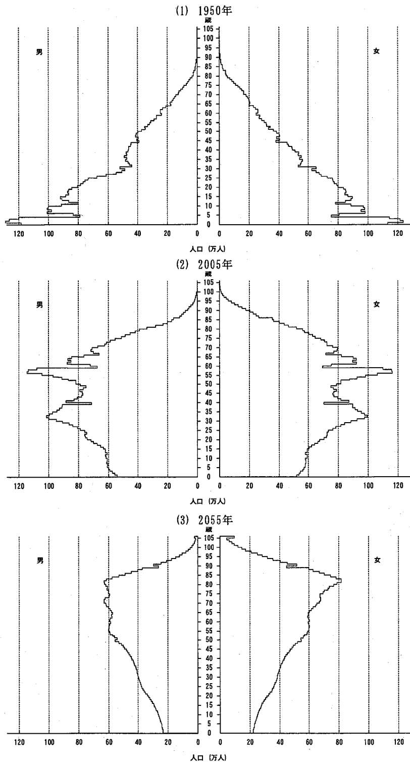
図2-1 人口ピラミッド：1950, 2005, 2055年
