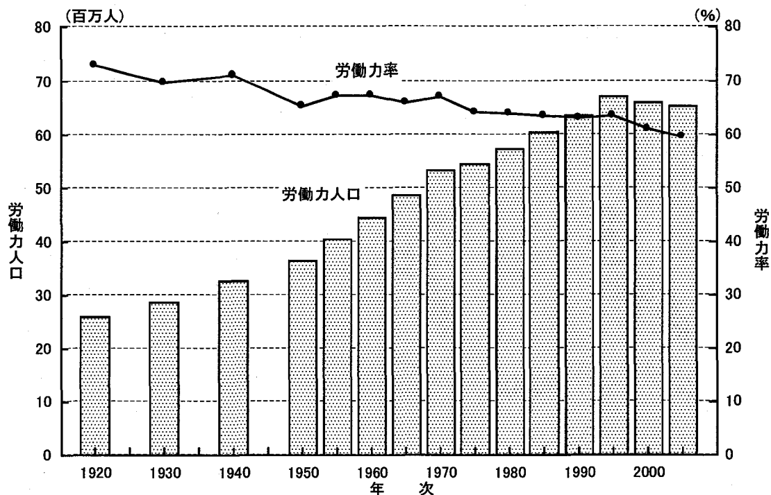
図 8 - 1 労働力人口および率：1920～2005年
