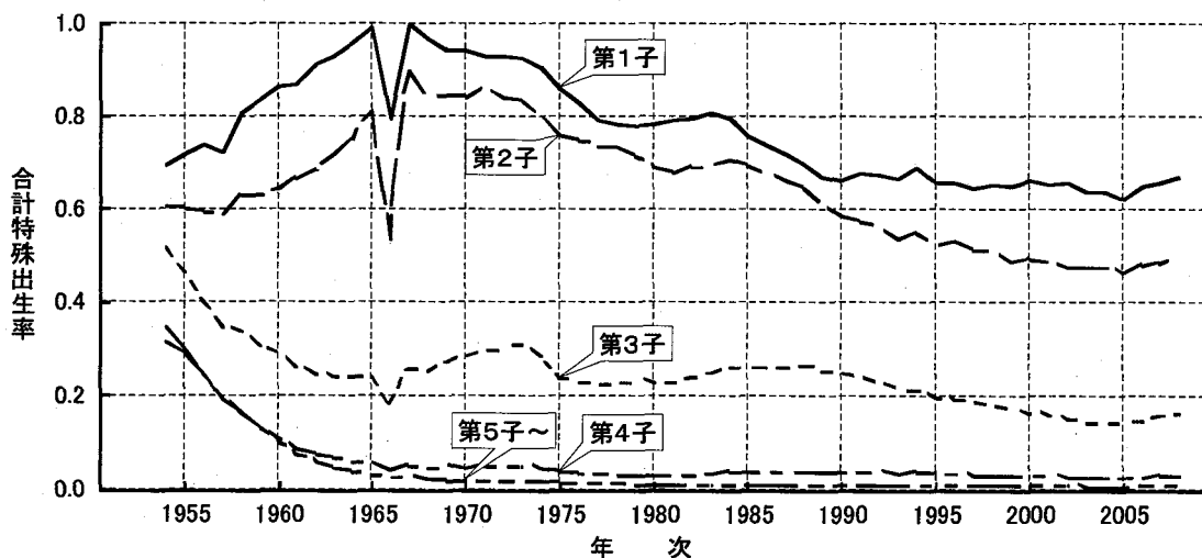
図4-6 出生順位別合計特殊出生率：1954～2008年
