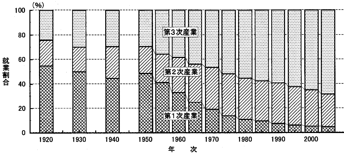
図8-6 産業(3部門)別就業割合:1920~2005年
