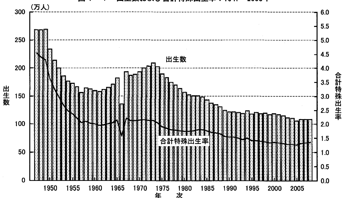
図4-1 出生数および合計特殊出生率：1947～2008年
