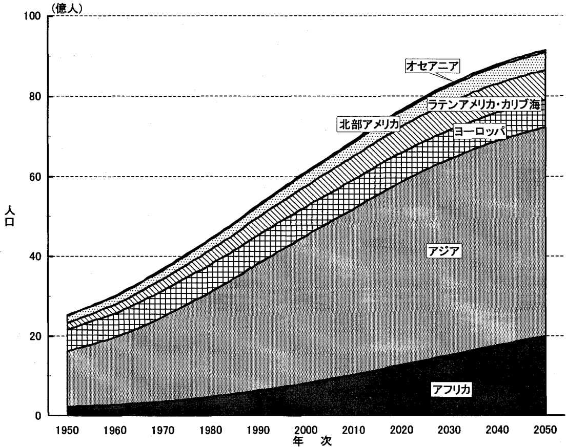
図 1 - 3 主要地域別人口：1950～2050年
