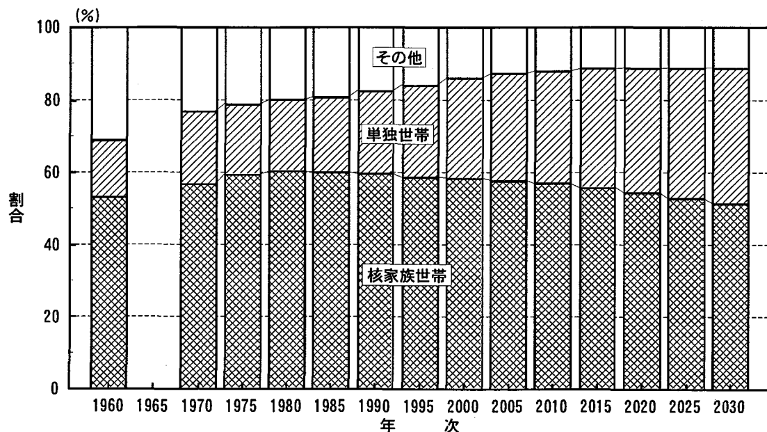
図7-2 一般世帯の家族類型別割合：1960～2030年
