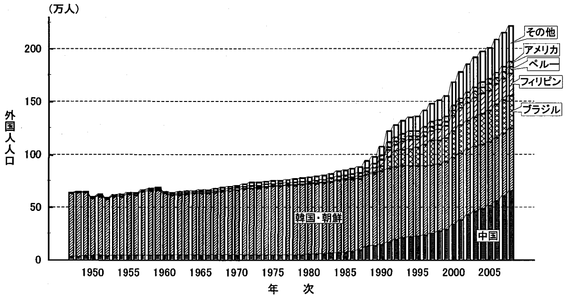
図10-1 国籍別登録外国人人口：1950～2008年
