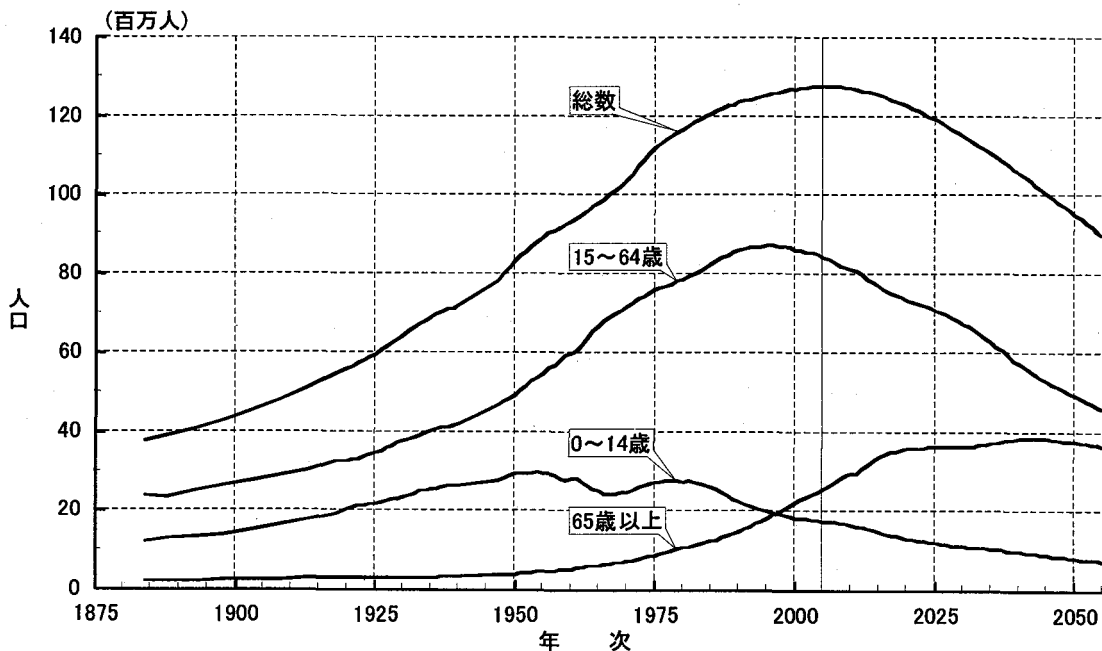
図2-2 年齢3区分別人口: 1884~2055年
