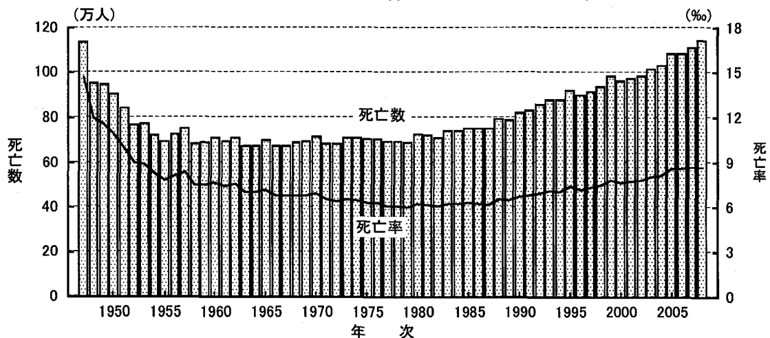
図5-1 死亡数および普通死亡率：1947～2008年
