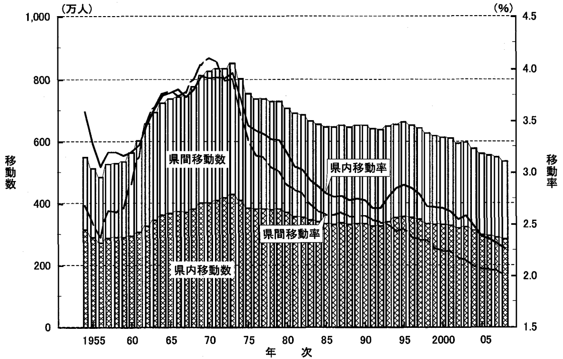
図9-1 県内・県間別人口移動数および率：1954~2008年
