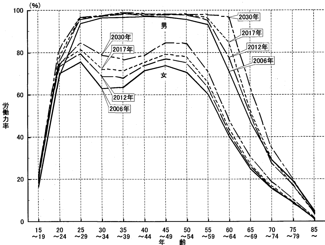
図8-3 性、年齢別労働力率の将来推計：2006～30年
