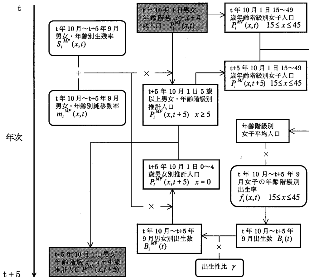
図1 コーホート要因法による都道府県別人口推計の手順
